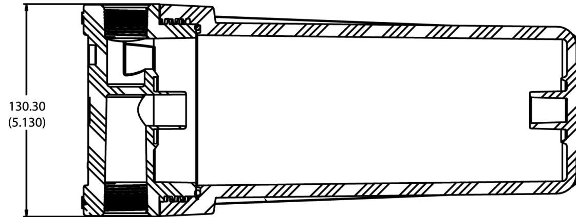
SECTION A-A
